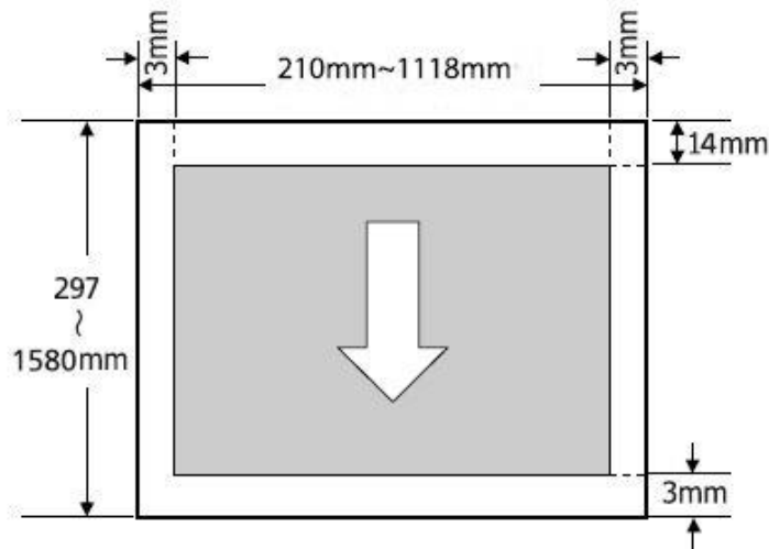
Skizze: Minimale Druckränder bei Blattware
